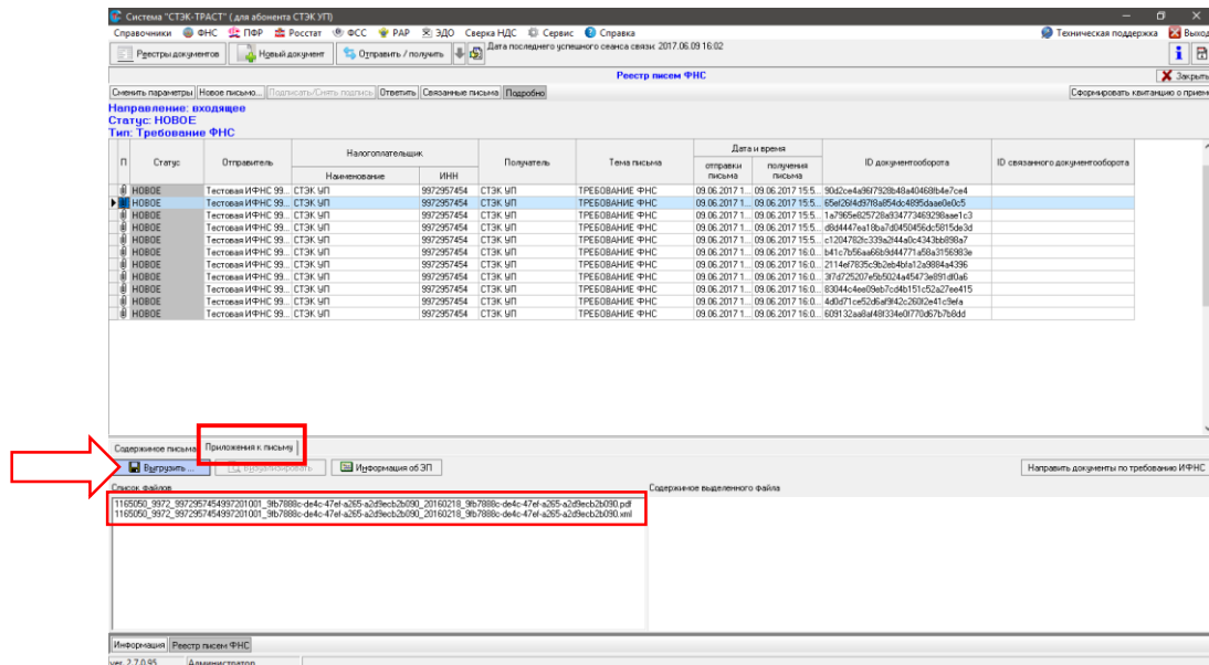
Рис. 1. Выгрузка требования
